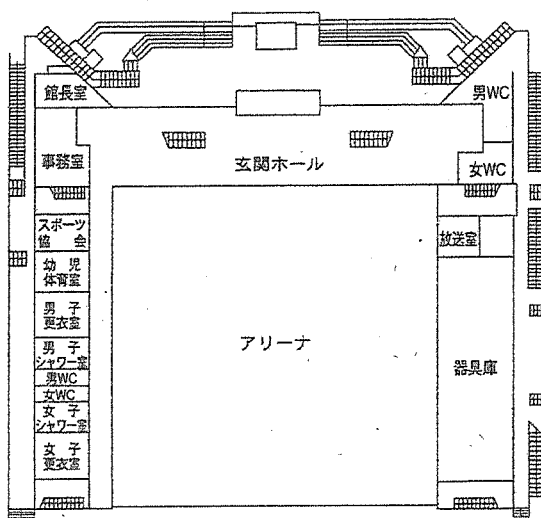
1階平面図
