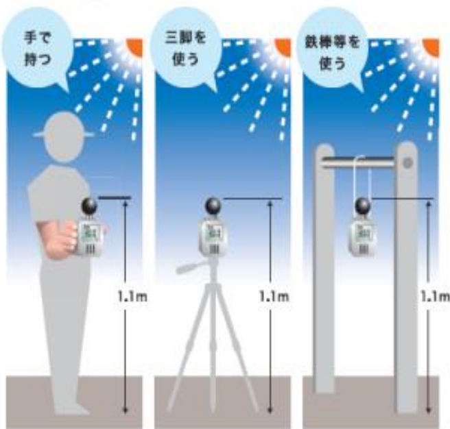
図1-5 暑さ指数 (WBGT) 計の使い方 (環境省：屋外日射の暑さ指数 (WBGT) 計の使い方)
